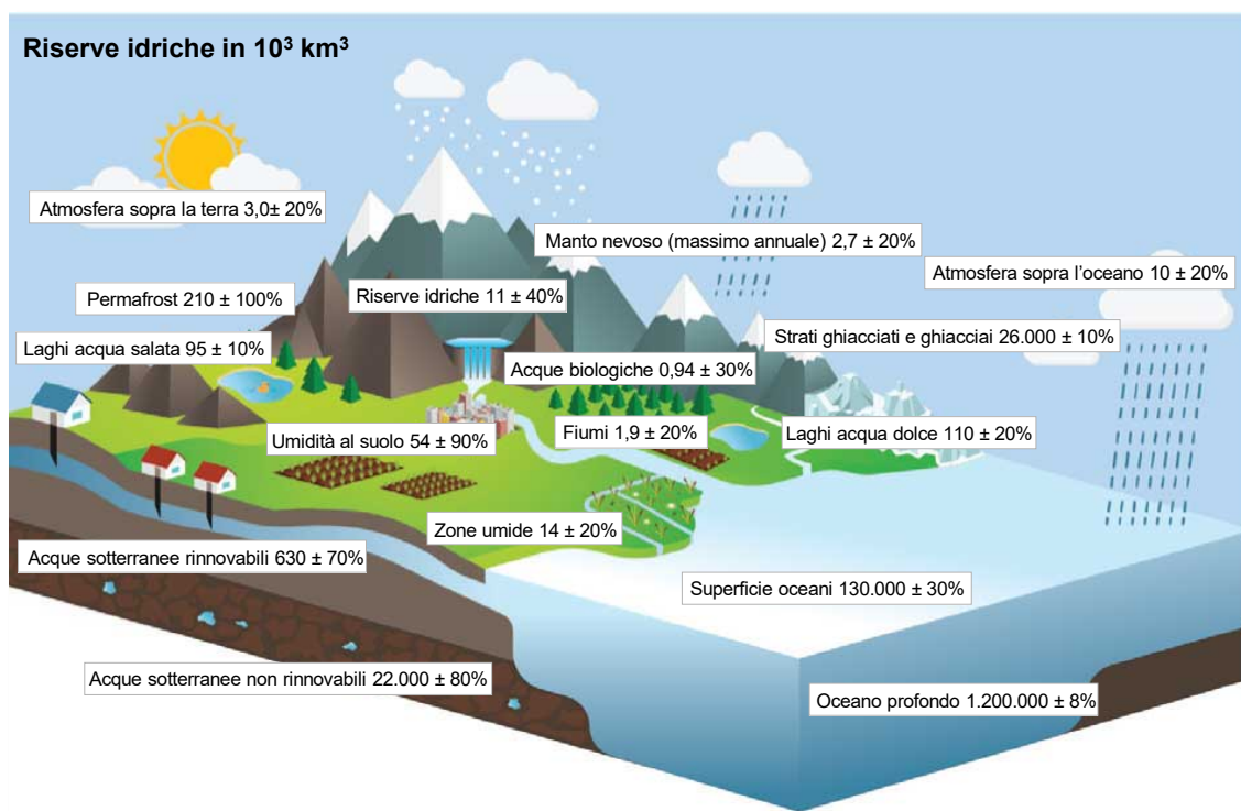
Figura 2. Ciclo idrogeologico globale nell'Antropocene con quantificazione delle riserve idriche e identificazione dei relativi comparti (modificato da UNESCO, 2020)
