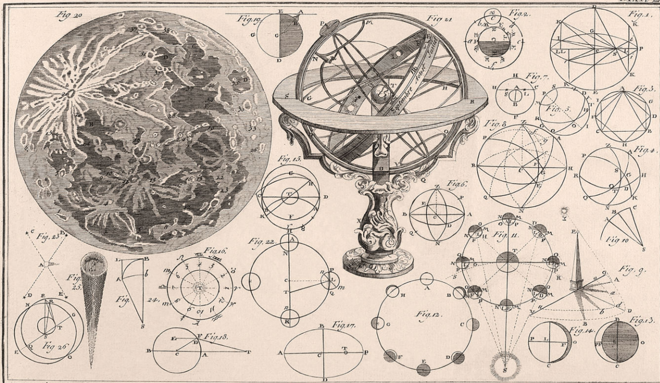
Astronomie.
