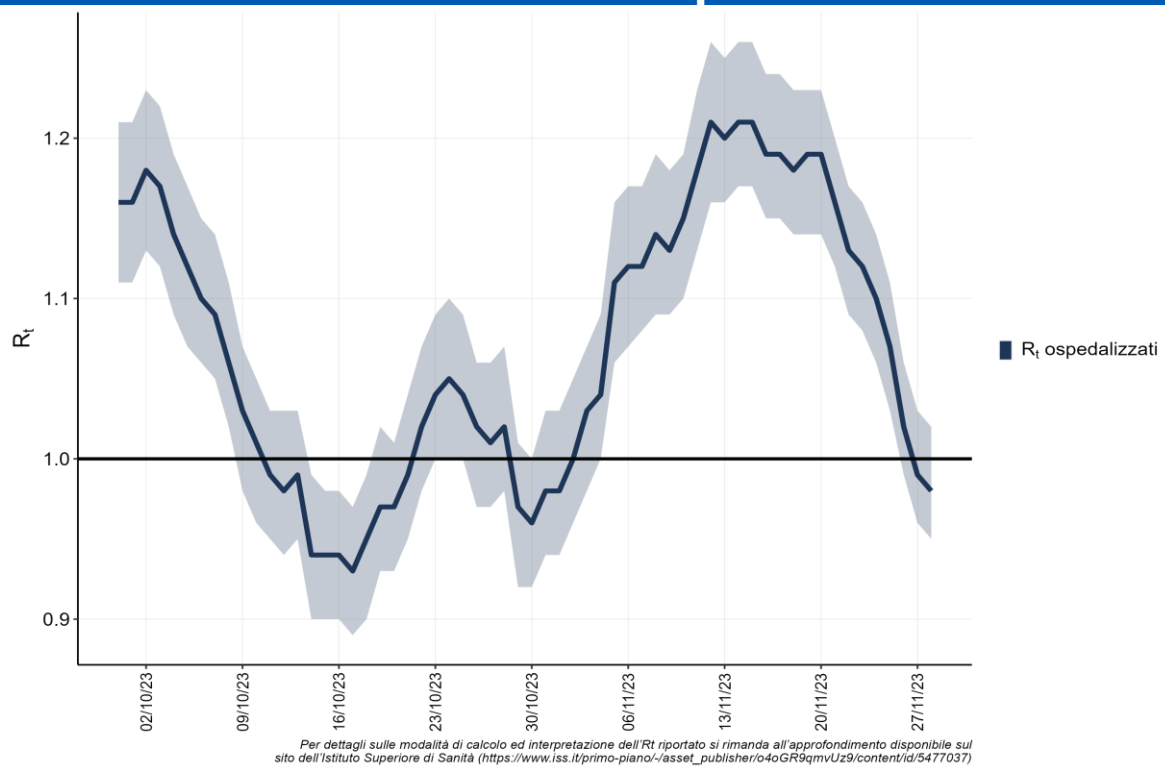
Figura 6 - Andamento giornaliero di Rt ospedalizzazioni nazionale, calcolato con dati estratti il 06 dicembre 2023
