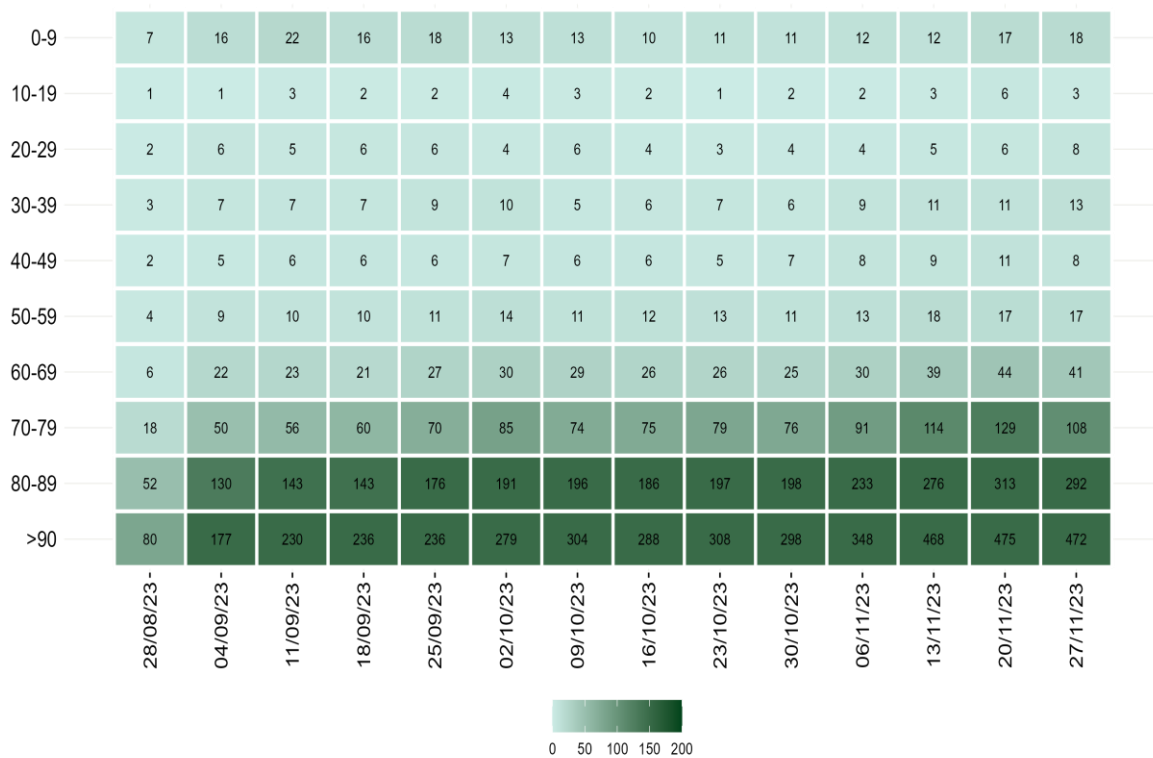
Figura 3 - Tasso di ospedalizzazione settimanale (per 1.000.000 ab.) per fascia d'età dal 28 agosto 2023
