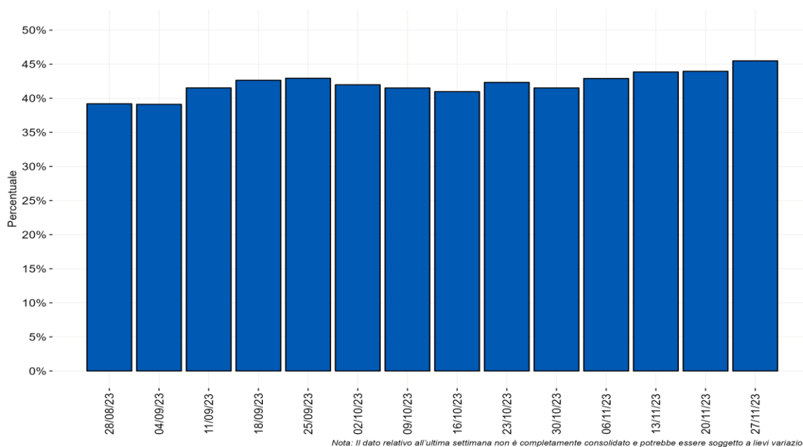
Figura 8 - Distribuzione percentuale settimanale delle diagnosi di reinfezione da SARS-CoV-2 sul totale delle diagnosi segnalate per data di prelievo/diagnosi a partire dal 28 agosto 2023
