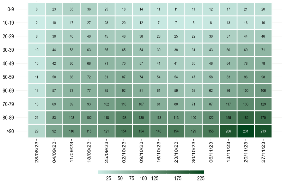
Figura 7 - Incidenza settimanale di infezioni da SARS-CoV-2 per 100.000 abitanti per fascia d'età, a partire dal 28 agosto 2023
