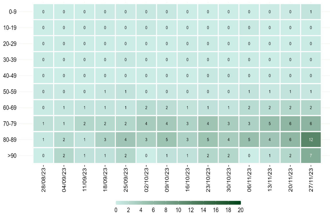
Figura 4 - Tasso settimanale di ricovero in terapia intensiva (per 1.000.000 ab.) per fascia d'età partire dal 28 agosto 2023
