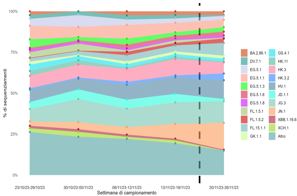
Figura 10 - Percentuale (%) dei principali sotto-lignaggi di SARS-CoV-2 per settimana di campionamento (periodo dal 23 ottobre al 26 novembre 2023 dati aggiornati al 4 dicembre 2023)
