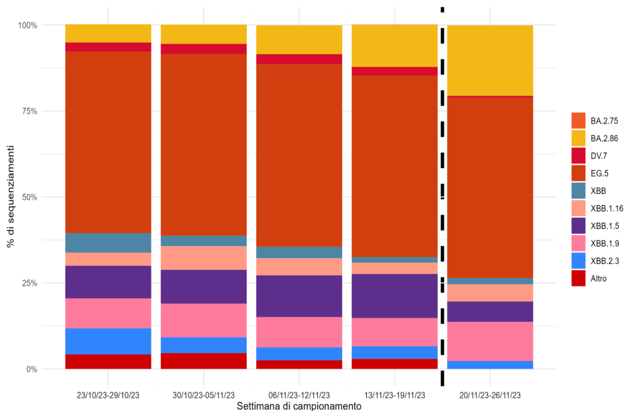
Figura 9 - Percentuale (%) dei principali lignaggi di SARS-CoV-2 per settimana di campionamento (periodo dal 23 ottobre al 26 novembre 2023 dati aggiornati al 4 dicembre 2023)
