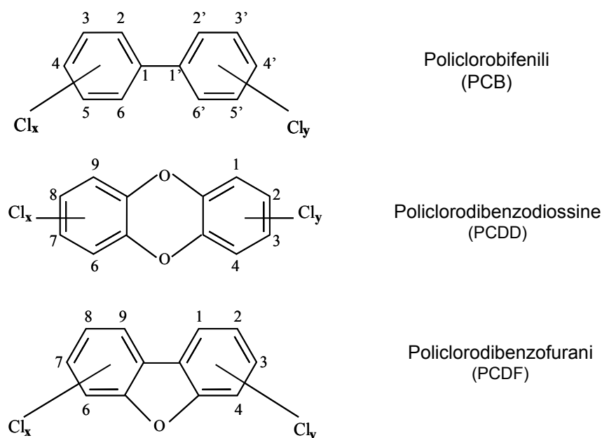
Figura 1. Formule di struttura dei PCB, PCDD e PCDF
