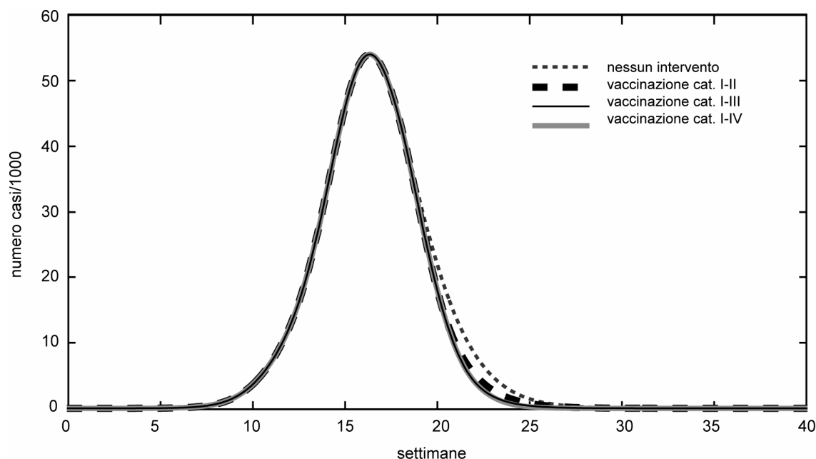
Figura 2. Impatto del vaccino pandemico
