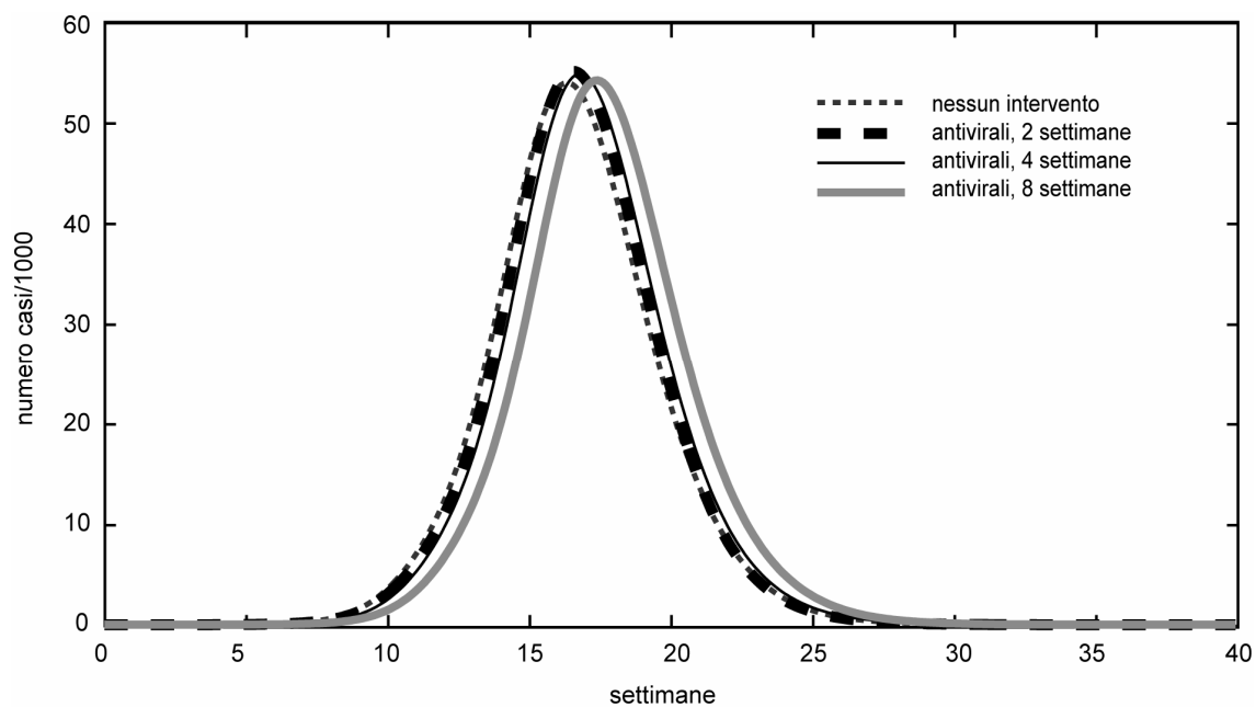
Figura 4. Impatto dell'uso di antivirali
