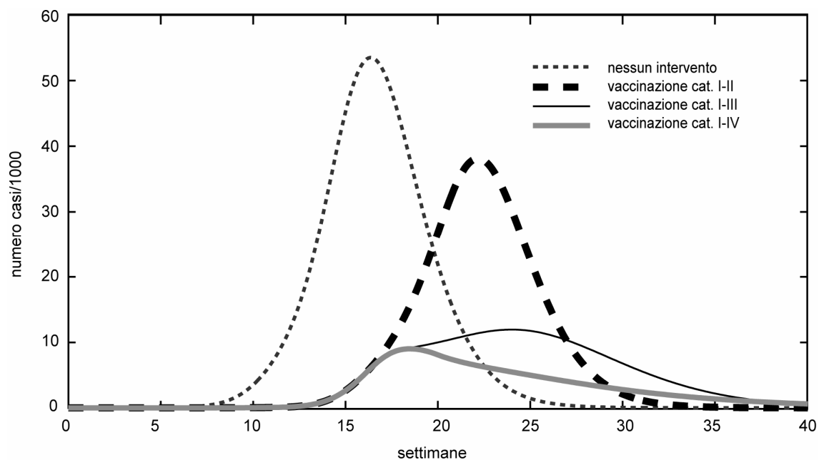
Figura 7. Impatto dell'uso associato di vaccino pre-pandemico, profilassi con antivirali per 8 settimane, e quarantena a partire dalla quarta settimana
