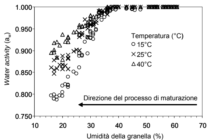
Figura 2. Isoterme di sorbimento a 15, 25, 40°C, per la granella di mais durante la maturazione
