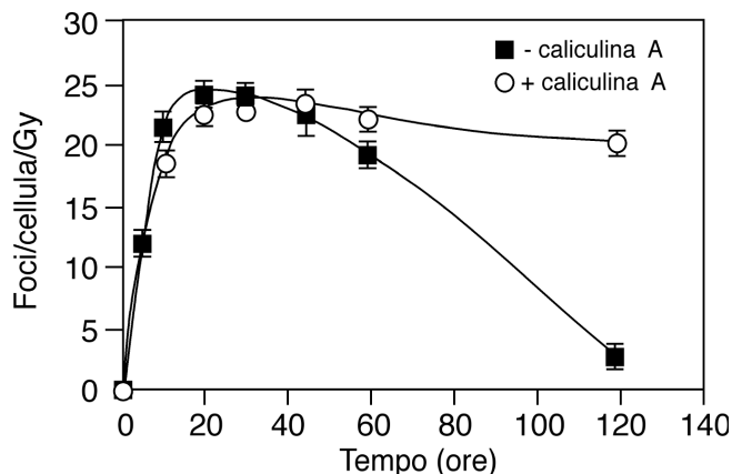
Figura 5. Cinetiche di fosforilazione-defosforilazione dell'istone H2AX dopo irraggiamento con 1 Gy di raggi gamma. Le cellule sono state successivamente incubate in assenza o in presenza di caliculina A. Le barre d'errore rappresentano l'errore standard sulla media di almeno 3 esperimenti. Non è stata fatta alcuna sottrazione del numero di foci del controllo (circa 0,08 foci/cell/Gy)
