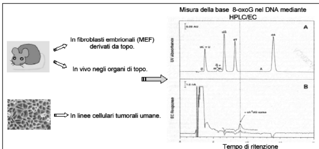
Figura 2. Misura dell'8-oxoG nel DNA mediante HPLC-EC
