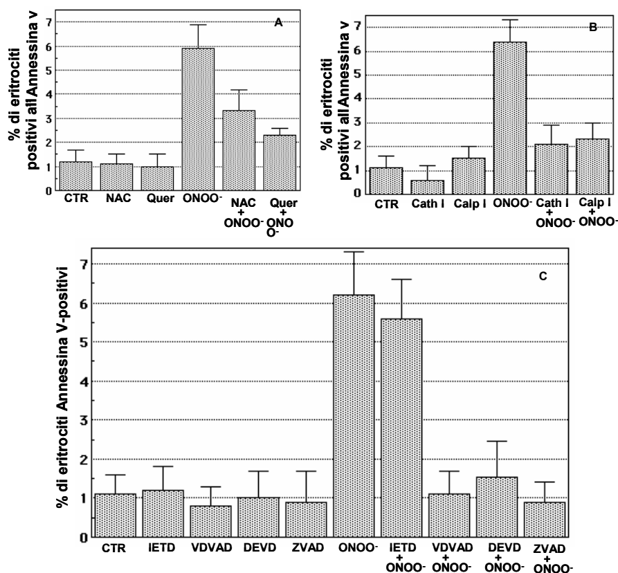
Figura 6. (A-C) Analisi citofluorimetrica dopo incubazione con annessina V-FITC per la rivelazione della PS sulla superficie degli eritrociti in diverse condizioni sperimentali
