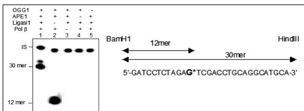
Figura 3. Ricostruzione in vitro della riparazione della 8oxoG (G*) con proteine purificate: autoradiografia di un gel denaturante di poliaccrilammide
