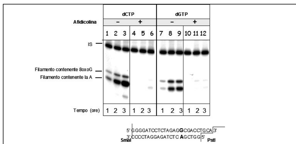
Figura 6. Cinetica di riparazione di 8-oxoG/A mediata da estratti cellulari di HeLa in presenza di afidicolina: autoradiografia di un gel di poliacrilamide denaturante.
