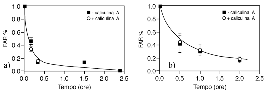
Figura 6. Cinetiche di ricongiungimento delle doppie rotture indotte nel DNA ottenute mediante analisi della FAR (24). Le barre d'errore rappresentano l'errore standard sulla media di 2 esperimenti
