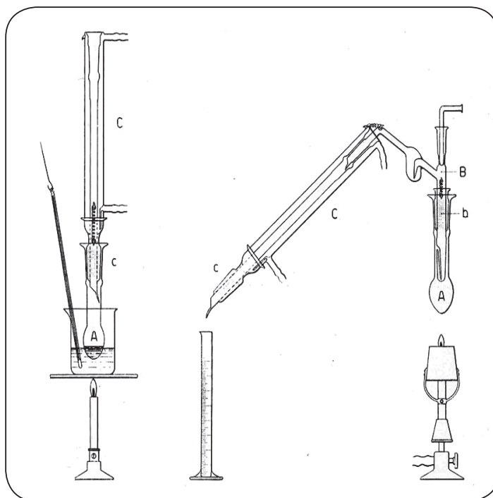
Figura 14. - Schema dell'apparecchio per la microdeterminazione del gruppo acetile e C-metile secondo Wiesener.
