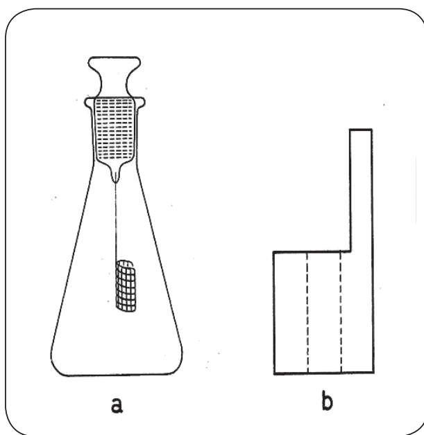
Figura 11. - Beuta e carta da filtro (o contenitore di cellulosa) per la combustione secondo Schöniger.
