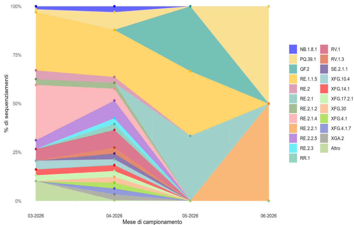
Figura 11 - Percentuale (%) dei principali sotto-lignaggi di SARS-CoV-2 per mese di campionamento
