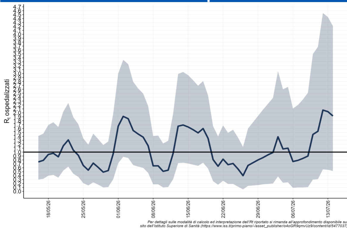
Figura 7 - Andamento giornaliero di R_t ospedalizzazioni nazionale, calcolato con dati estratti il 22 luglio 2026
