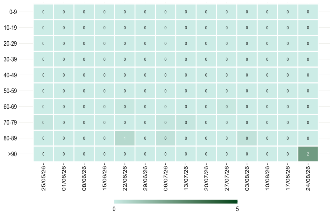
Figura 5 - Tasso settimanale di mortalità (per 1.000.000 ab.) per fascia d'età a partire dal 25 maggio 2026
