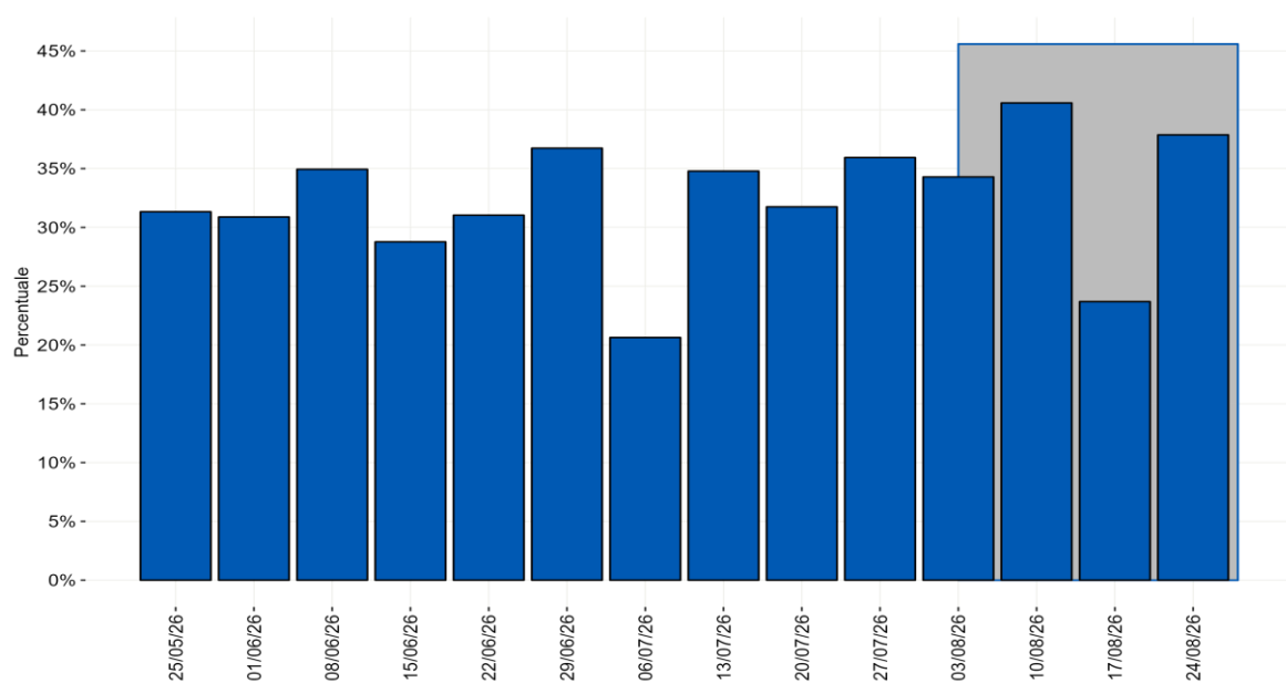
Figura 8 - Distribuzione percentuale settimanale delle diagnosi di reinfezione da SARS-CoV-2 sul totale delle diagnosi segnalate per data di prelievo/diagnosi a partire dal 25 maggio 2026
