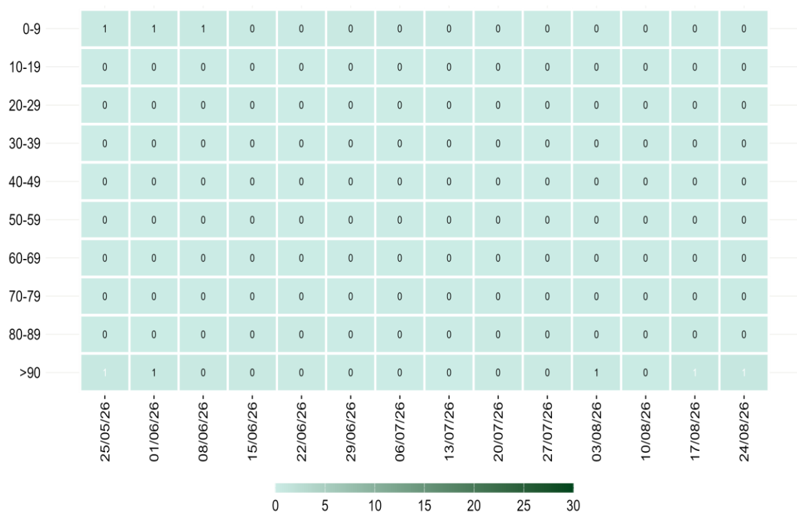
Figura 7 - Incidenza settimanale di infezioni da SARS-CoV-2 per 100.000 abitanti per fascia d'età, a partire dal 25 maggio 2026
