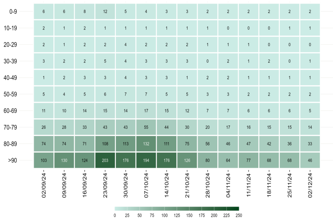
Figura 3 - Tasso di ospedalizzazione settimanale (per 1.000.000 ab.) per fascia d'età dal 2 settembre 2024
