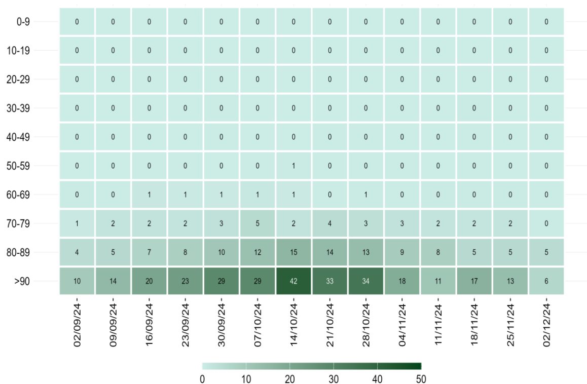
Figura 5 - Tasso settimanale di mortalità (per 1.000.000 ab.) per fascia d'età a partire dal 2 settembre 2024
