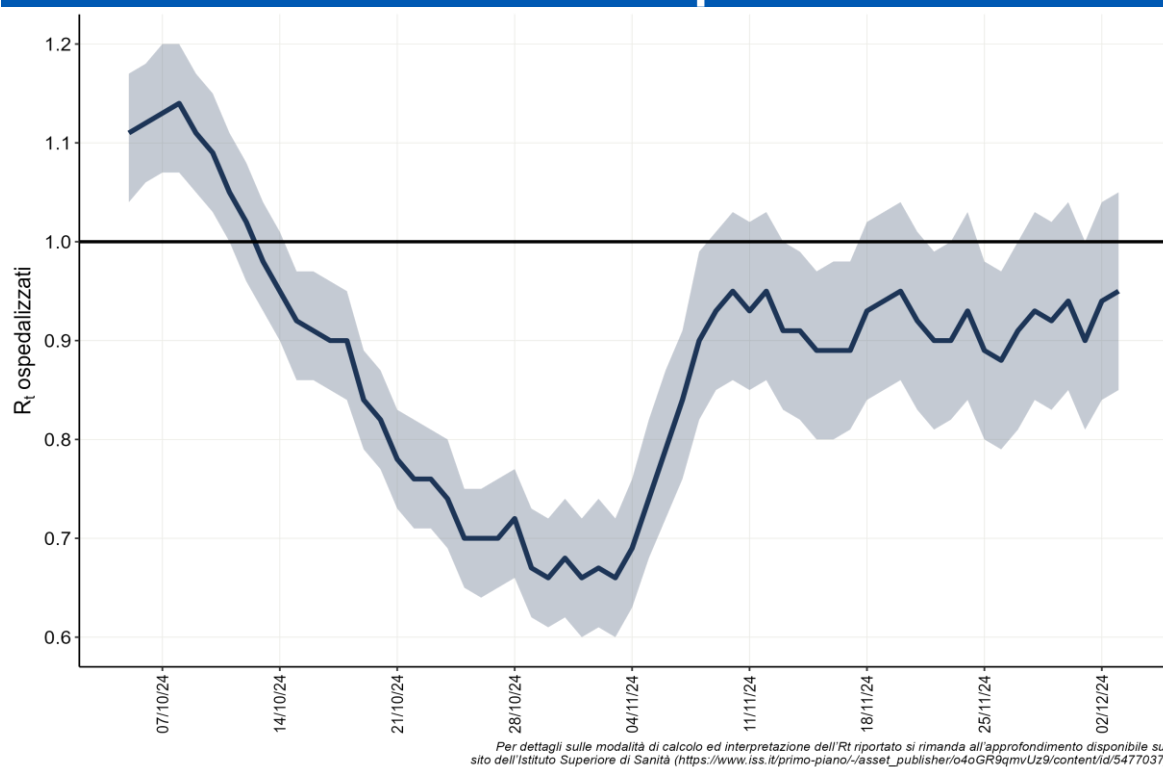
Figura 6 - Andamento giornaliero di Rt ospedalizzazioni nazionale, calcolato con dati estratti il 11 dicembre 2024
