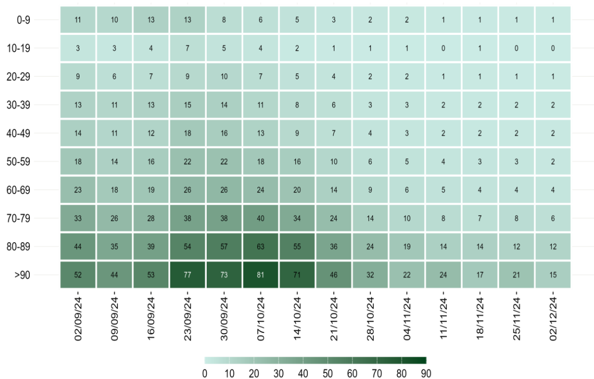
Figura 7 - Incidenza settimanale di infezioni da SARS-CoV-2 per 100.000 abitanti per fascia d'età, a partire dal 2 settembre 2024
