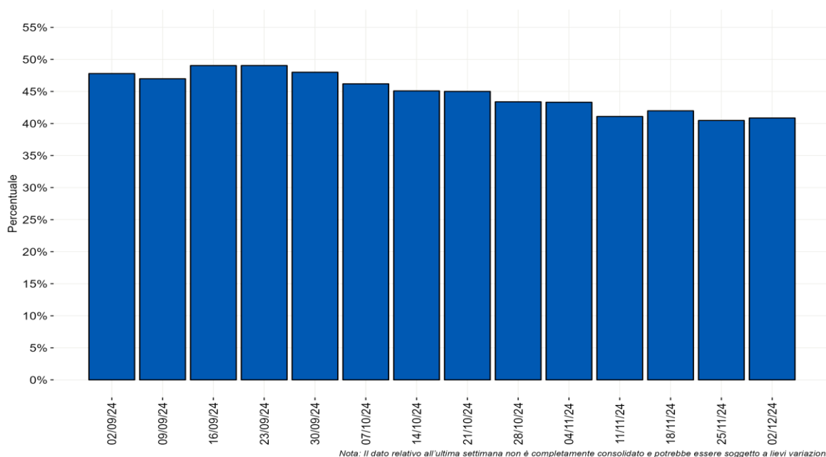
Figura 8 - Distribuzione percentuale settimanale delle diagnosi di reinfezione da SARS-CoV-2 sul totale delle diagnosi segnalate per data di prelievo/diagnosi a partire dal 2 settembre 2024
