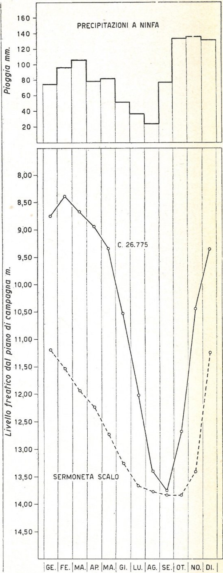
Rapporto tra le oscillazioni dei livelli acquiferi dei pozzi Casello 26775 e Sermoneta Scalo con le precipitazioni su Ninfa.
