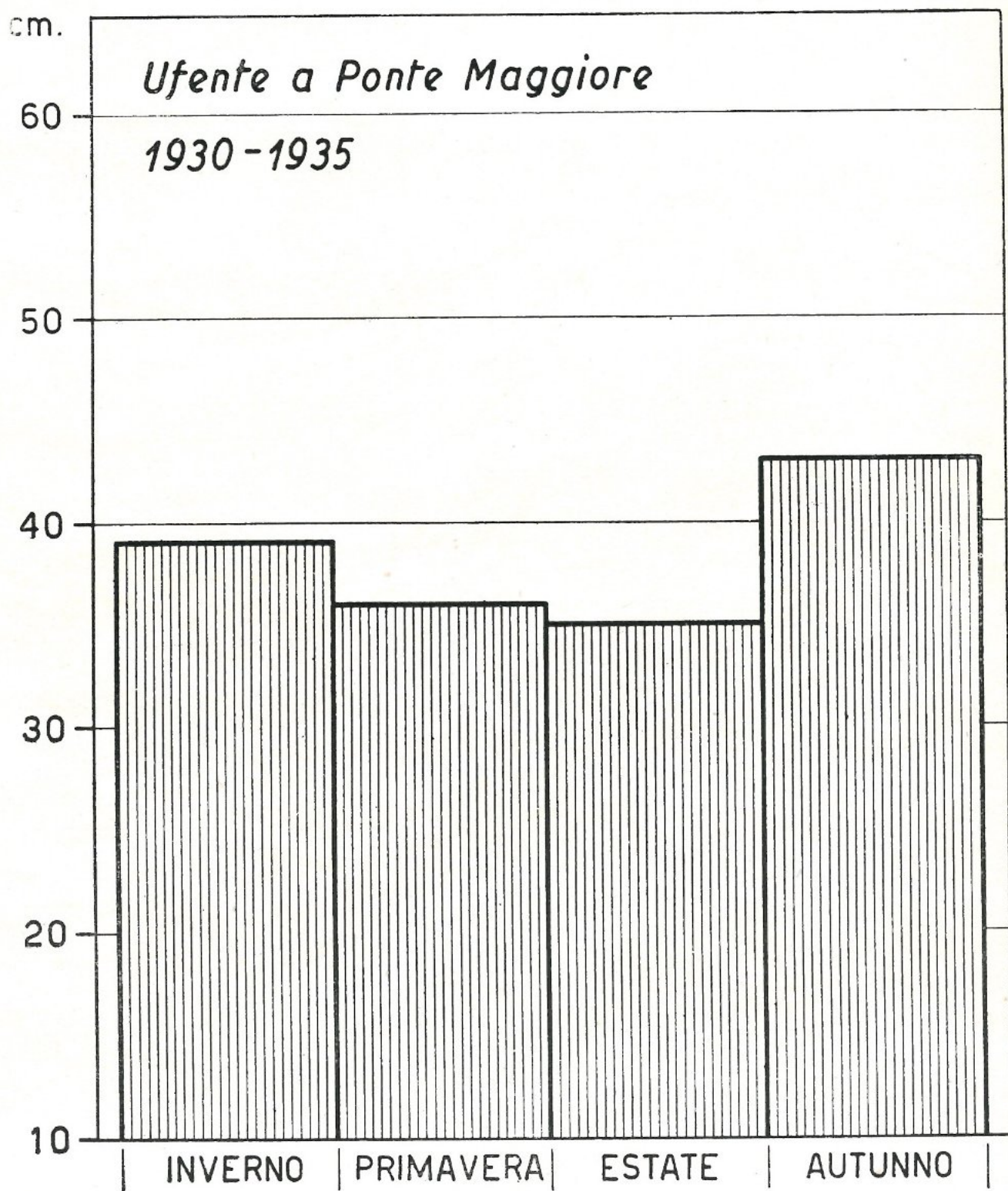
Medie stagionali delle altezze idrometriche del fiume Ufente a Ponte Maggiore nel periodo 1930-1935.
