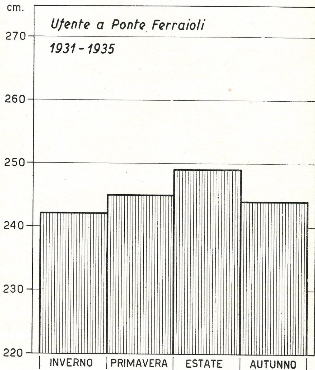
Medie stagionali delle altezze idrometriche del fiume Ufente a Ponte Ferraioli nel quinquennio 1931-1935.
