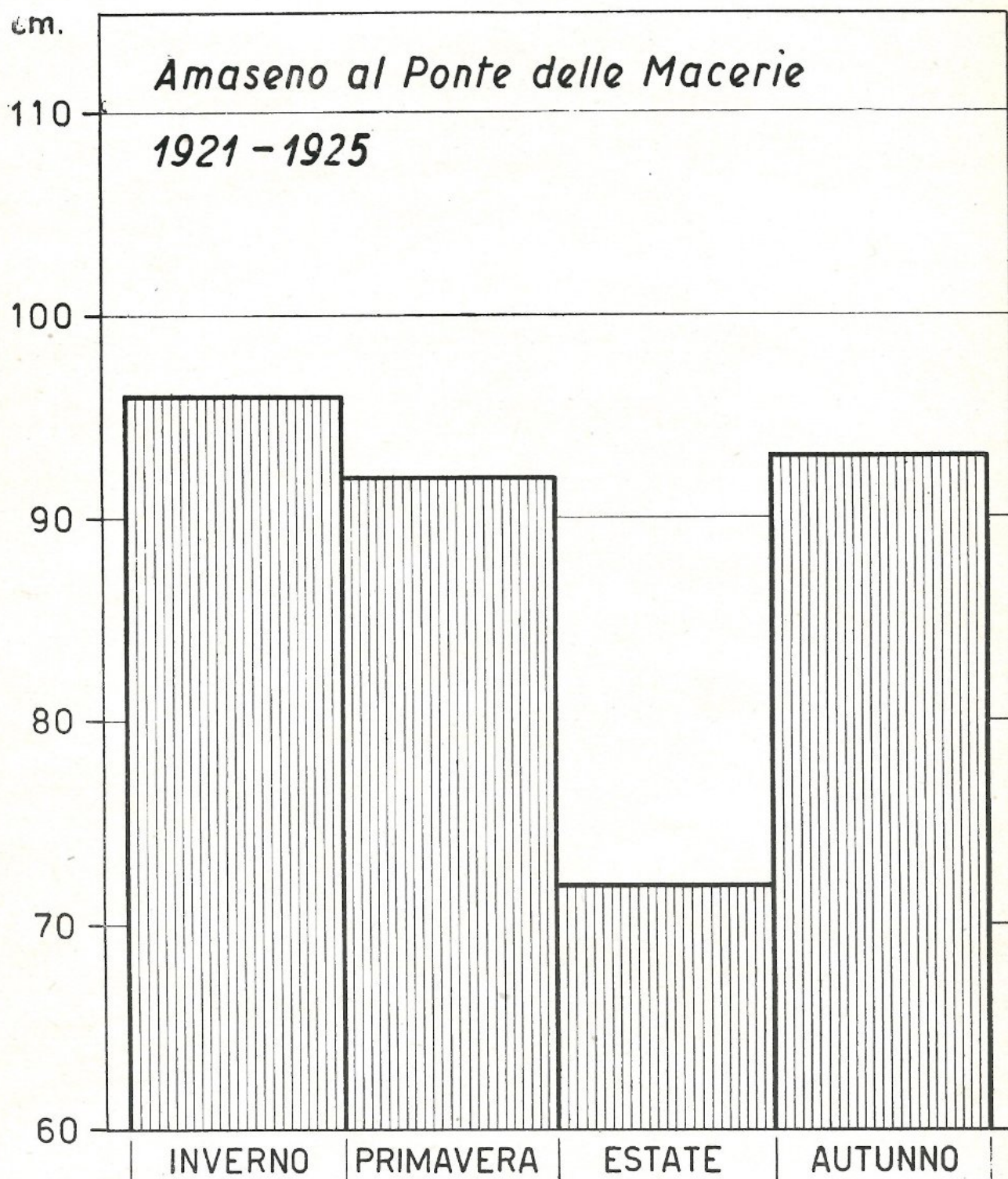
Medie stagionali delle altezze idrometriche del fiume Amaseno a Ponte delle Macerie nel quinquennio 1921-1925
