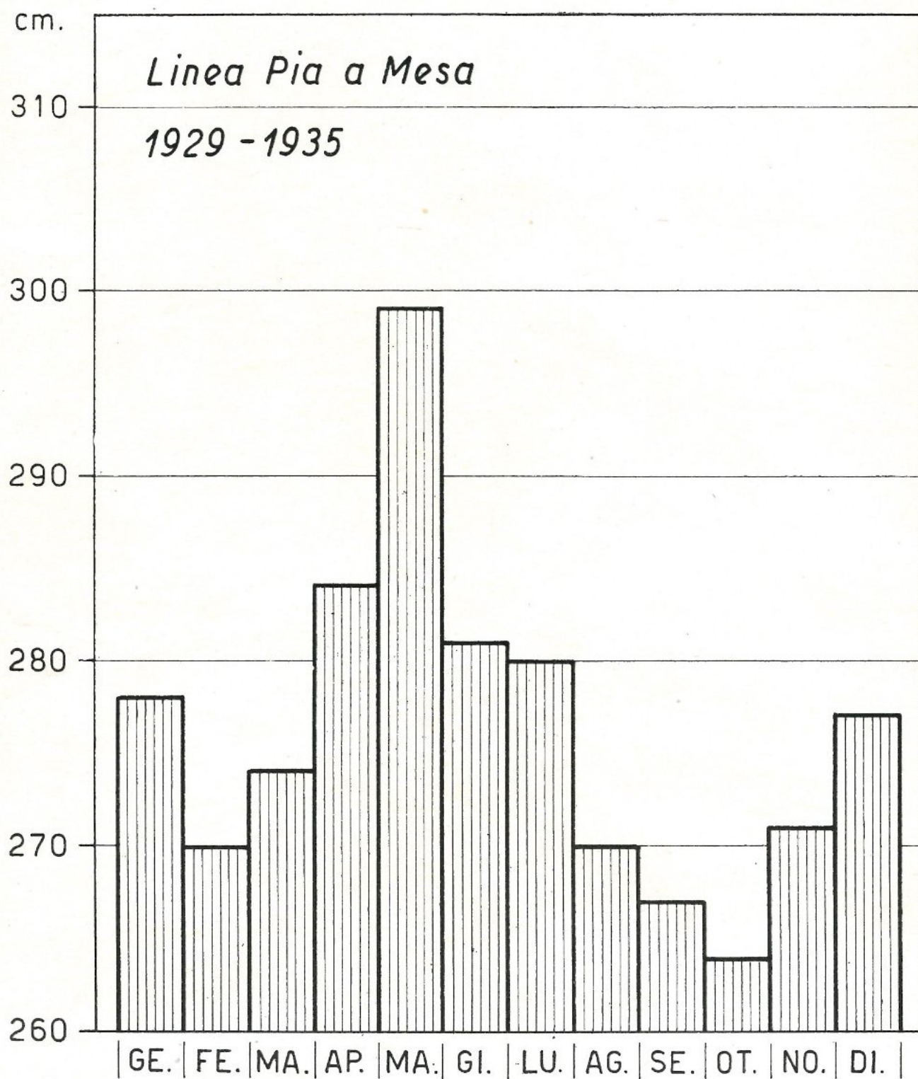
Medie mensili delle altezze idrometriche della Linea Pia a Mesa nel periodo 1929-1935.
