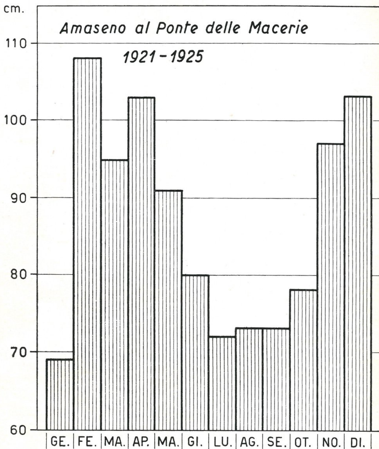
Medie mensili delle altezze idrometriche del fiume Amaseno al Ponte delle Macerie nel quinquennio 1921-1935.
