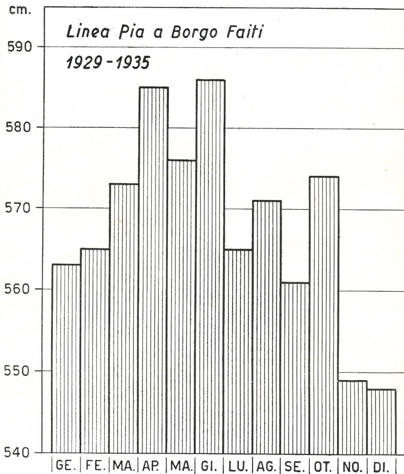
Medie mensili delle altezze idrometriche della Linea Pia a Borgo Faiti nel periodo 1929-1935
