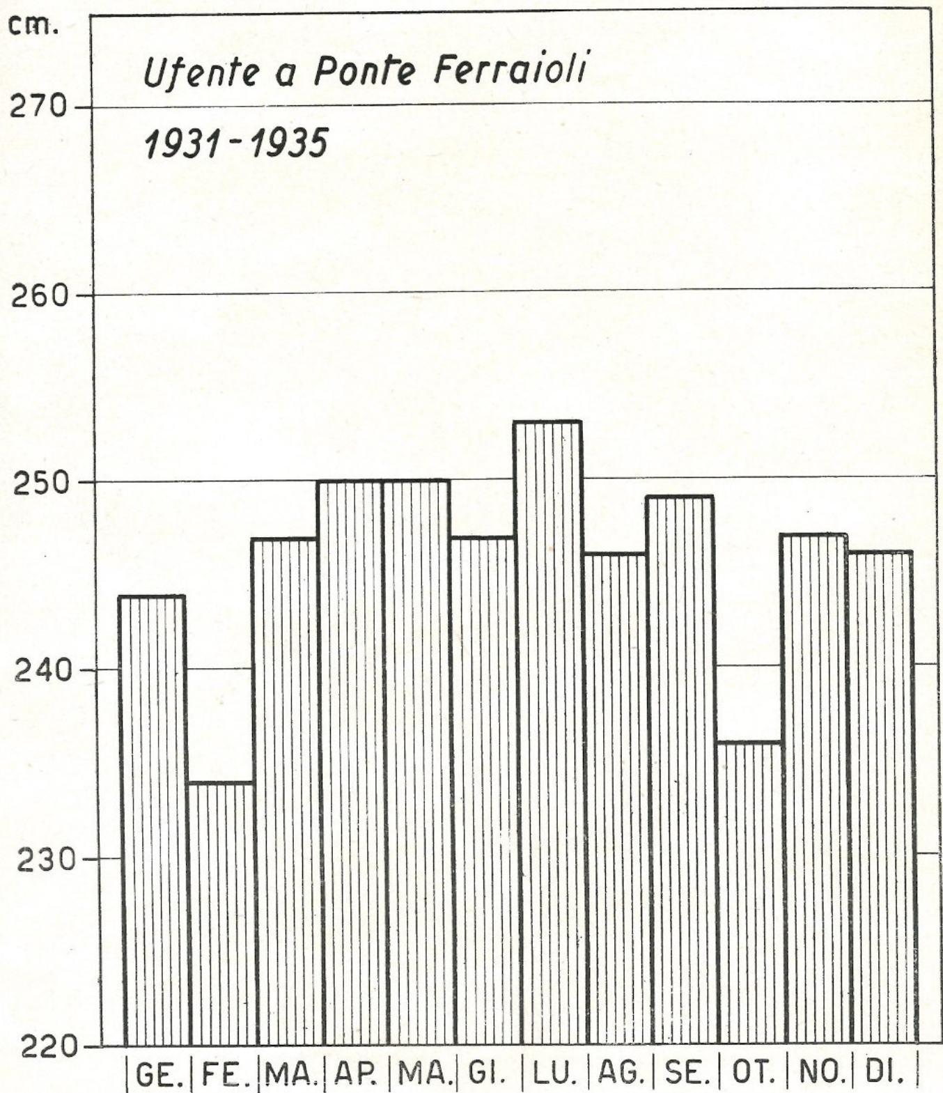
Medie mensili delle altezze idrometriche del fiume Ufente a Ponte Ferraioli nel quinquennio 1931-1935.
