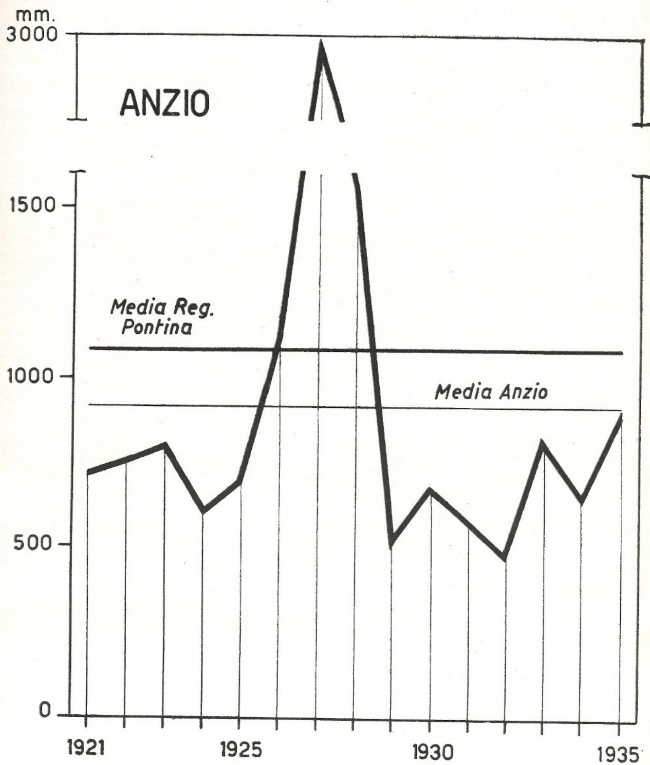
Totali annui delle precipitazioni su Anzio nel quindicennio 1921-1935.
