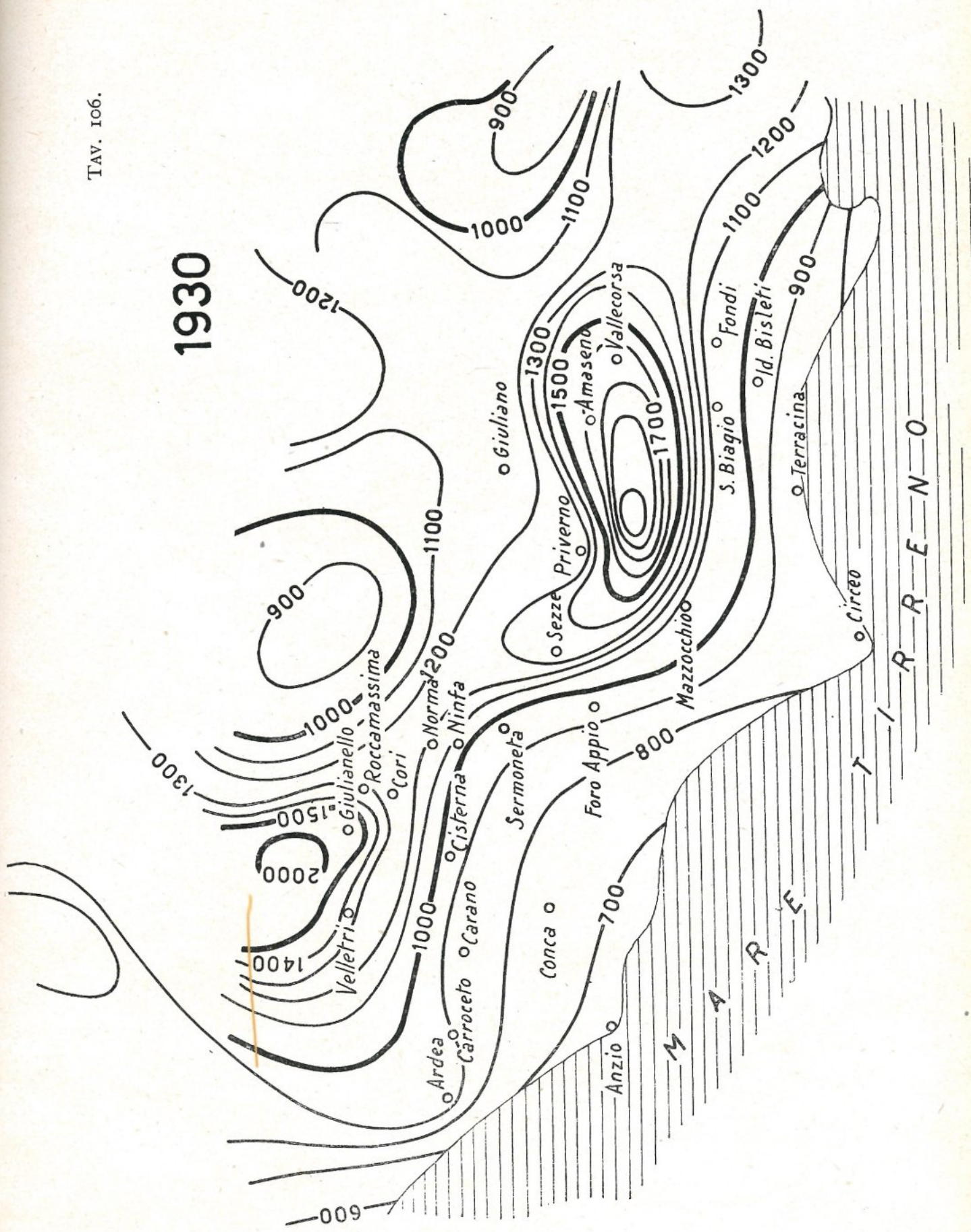
Carta delle isoiete per il 1930.
