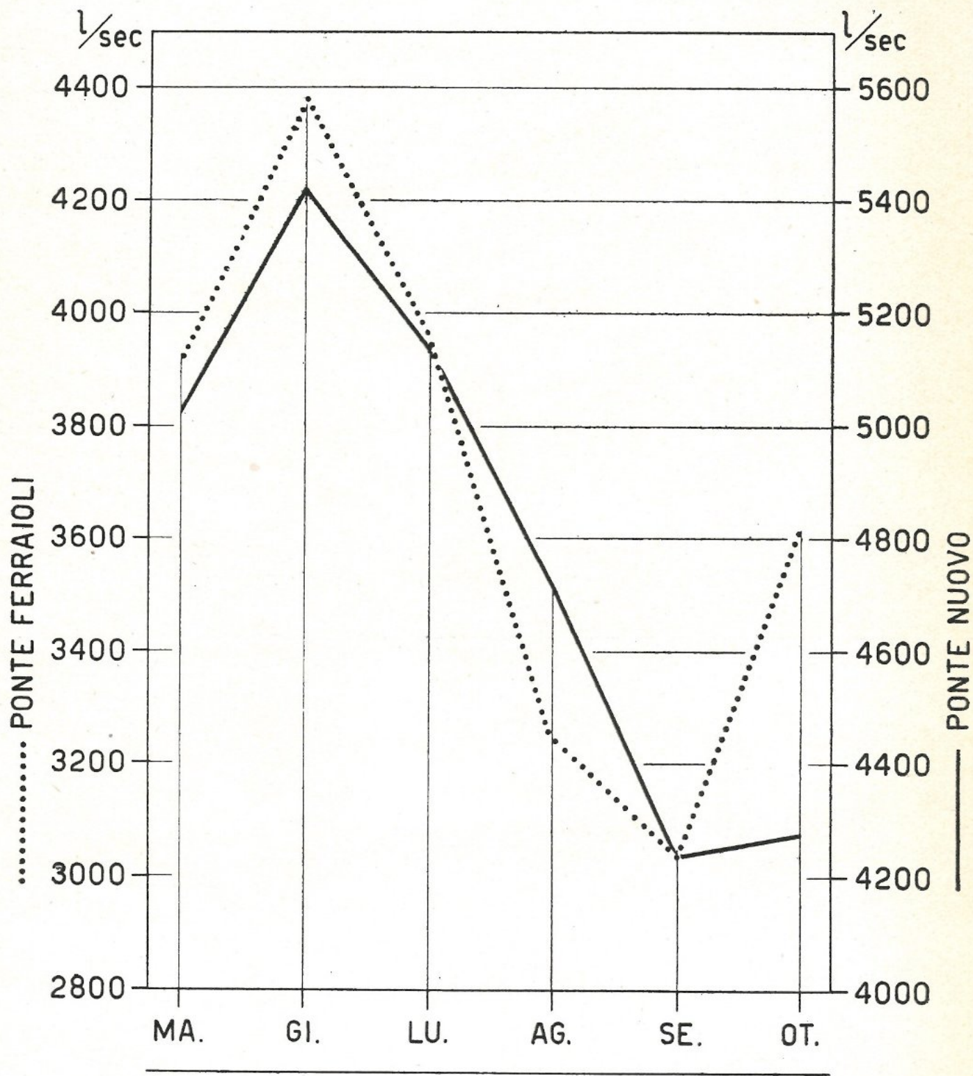
Portate minime mensili dell'Ufente a Ponte Ferraioli e a Ponte Nuovo.
