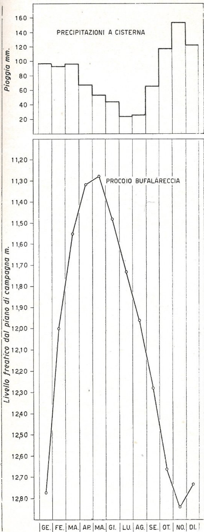
Rapporto tra le oscillazioni dei livelli acquiferi del pozzo di Procojo con le precipitazioni su Cisterna.
