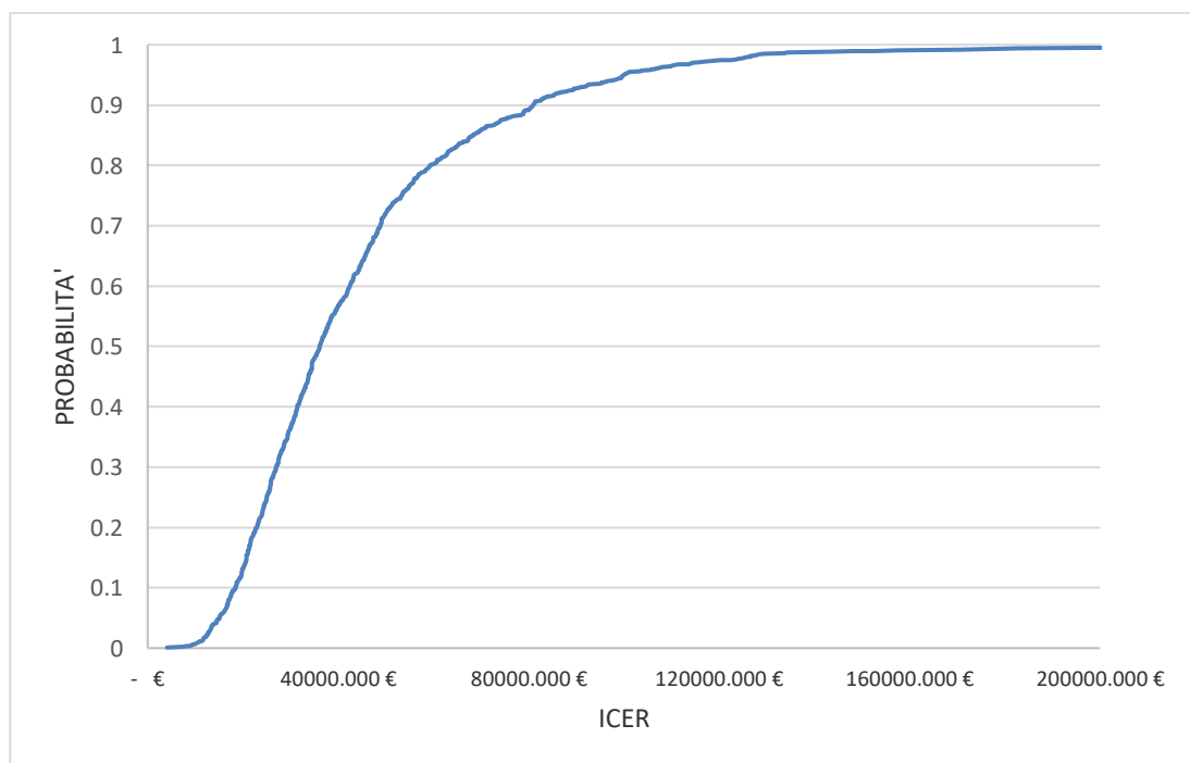
Figura 6. Pazienti ipotesi: curva di accettabilità del rapporto costo efficacia
